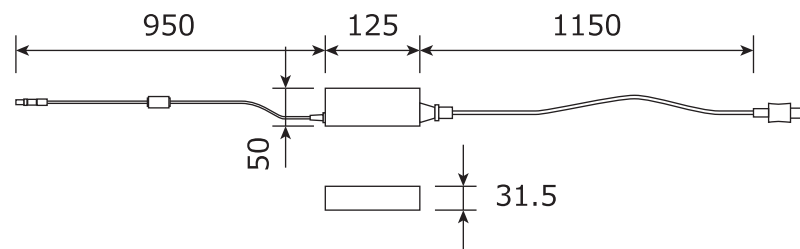
【アダプタ寸法】
